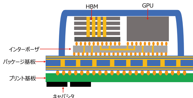
(図表1) 生成AI向け半導体の略図
