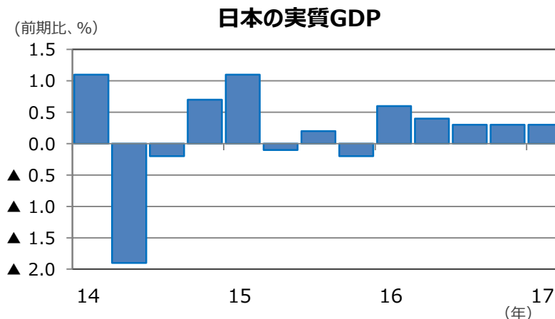
(注) データは2014年1-3月期～2017年1-3月期。 (出所) 内閣府などのデータを基に三井住友アセットマネジメント作成
